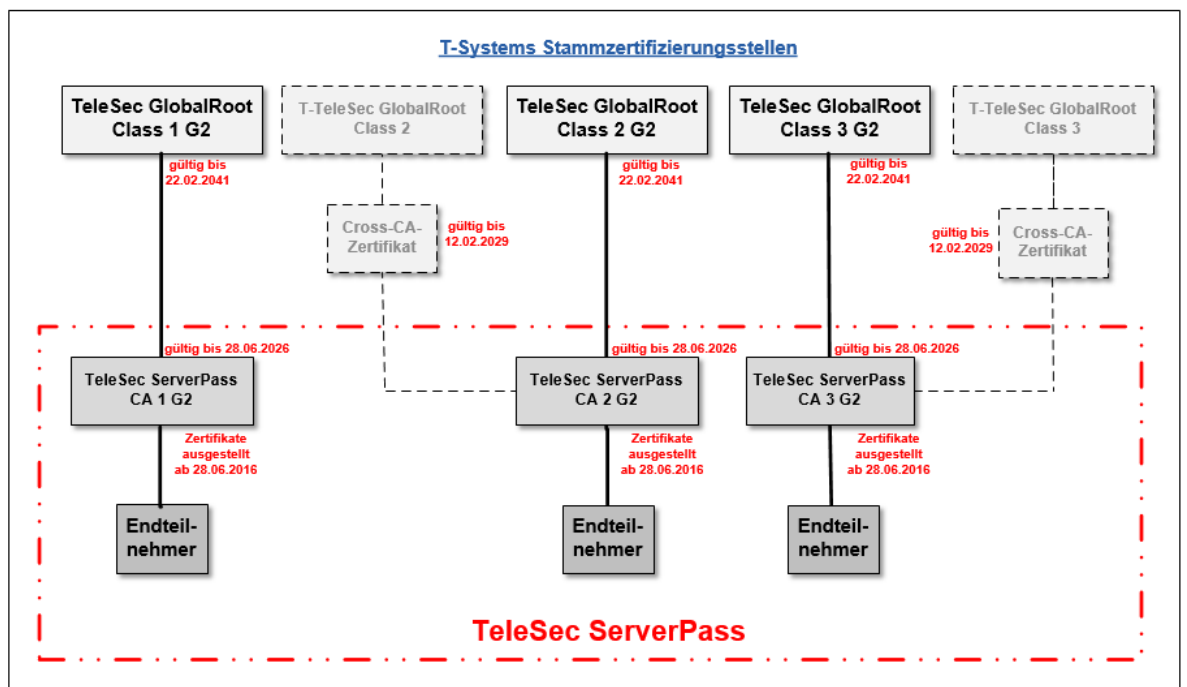
Abbildung 2: Übersicht der ECC-Zertifikathierarchien für TeleSec ServerPass
